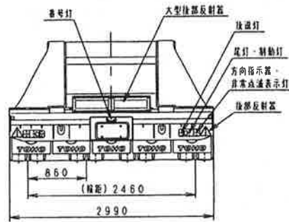
東邦TL50K0T2S型セミトレーラ外観四面図
